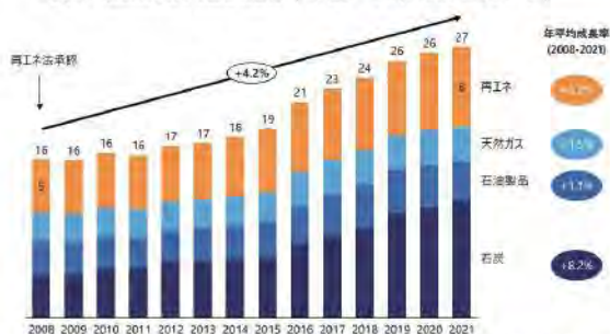
図1. 電源別導入容量推移（単位：GW, 2008-2021年）
